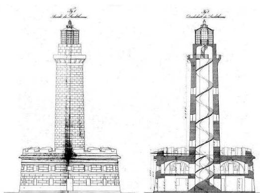
Progetto di Pietro Nobile per il Faro di Salvore
